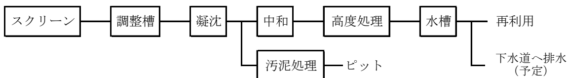
図 1-3.7(2) 無機系排水（ボイラ・ポンプ等機器冷却水・灰污水）の参考フロー例
