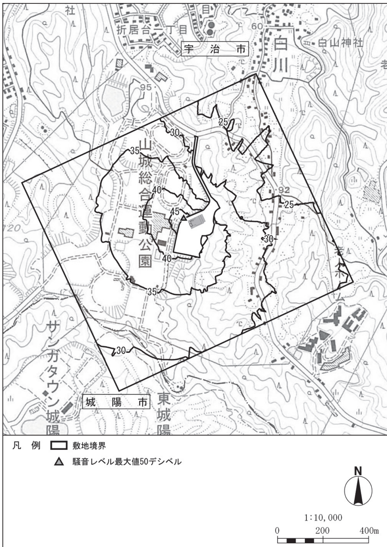
図 5-1-2.15 施設の稼働に伴う工場事業場騒音( L_{Aeq} )の予測結果 (朝・夕・夜間)
