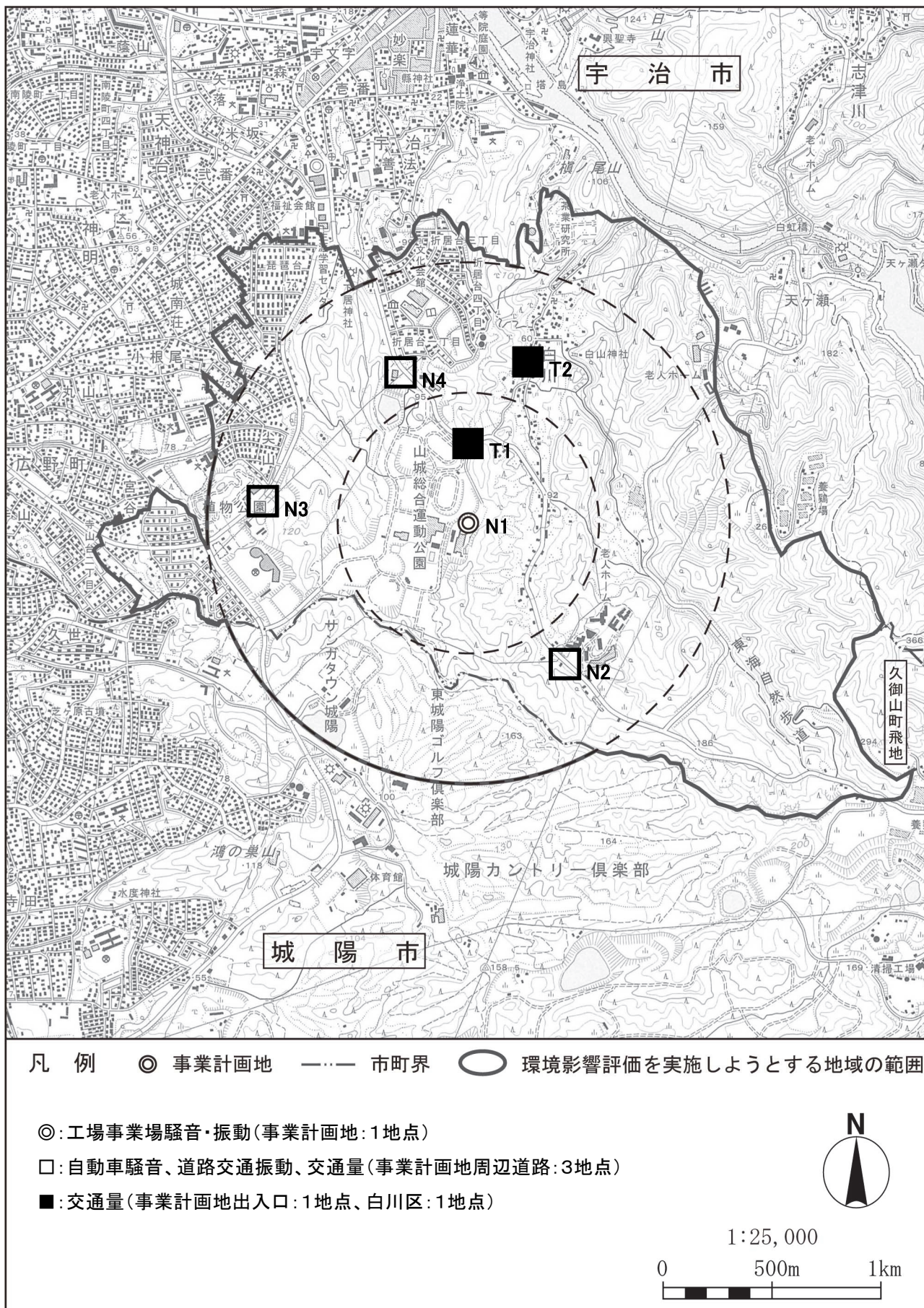
図 5-1-2.1 騒音・振動の現地調査地点
