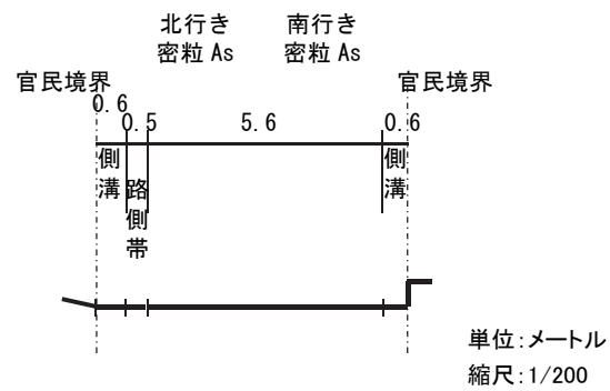
図 5-1-2.4(2) 道路断面図
