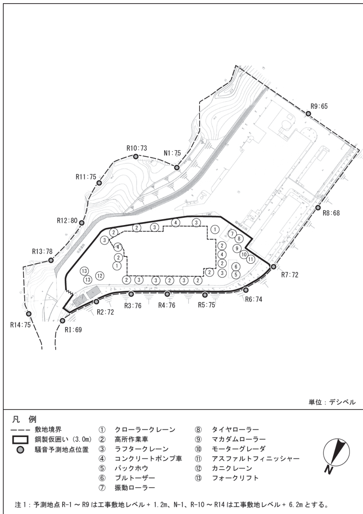
図 5-1-2.7 施設の建設工事に伴う建設作業騒音 ( L_{A5} ) の予測結果 (工事開始後 18 か月目)
